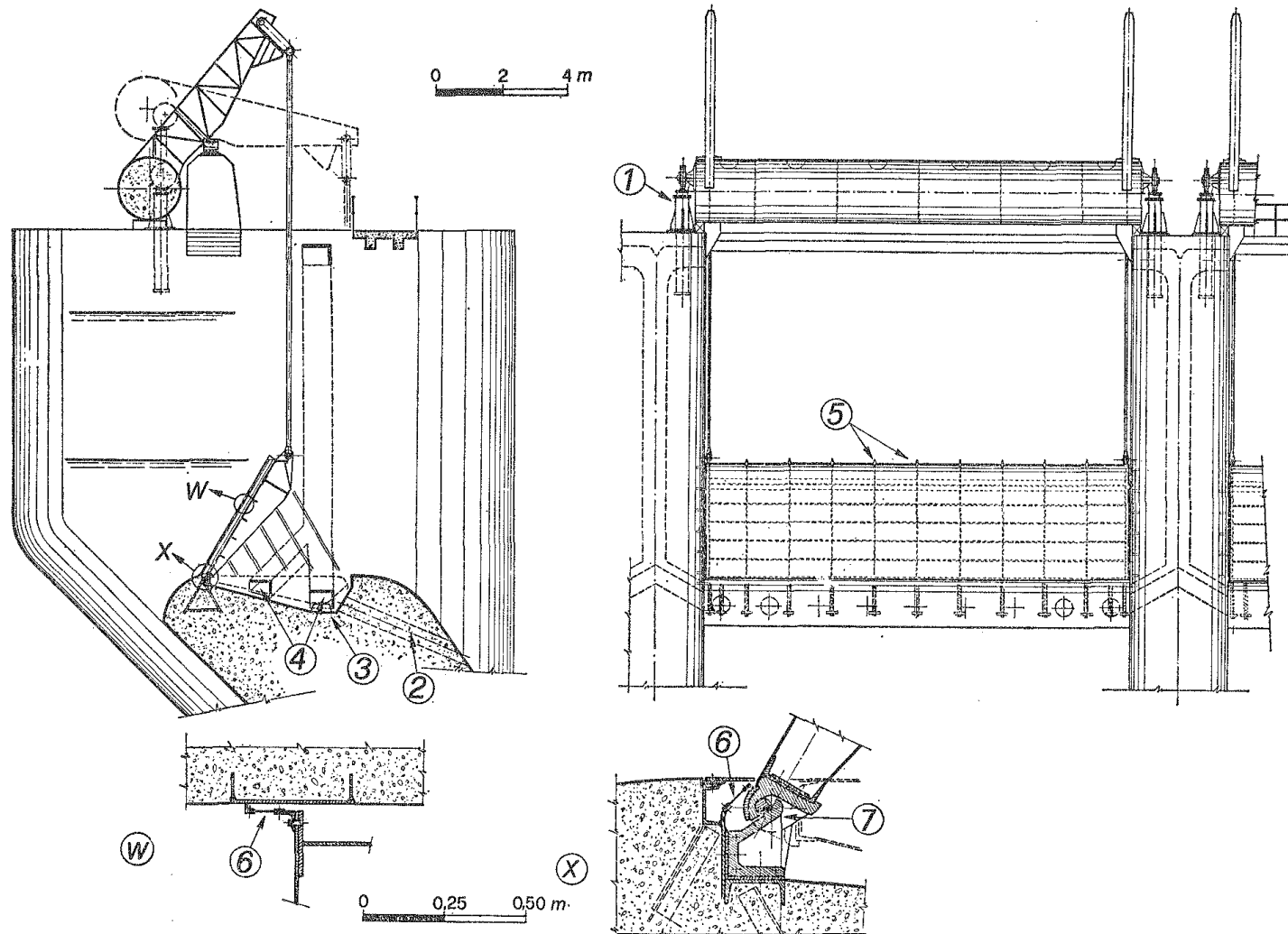
Fig. XVIII, 59. — Paratoia a ventola compensata automatica (A. CALZONI, Bologna). Sezione sull'asse della luce, prospetto da monte, dispositivi di tenuta laterale ( W ) e di monte ( X ). 1, Martineti per abbattimento volontario; 2, fori di scarico del cavo di alloggiamento; 3, zoccoli laterali di appoggio; 4, condotti di aereazione; 5, frangivena; 6, lamierini di tenuta; 7, cerniere a coltello.
