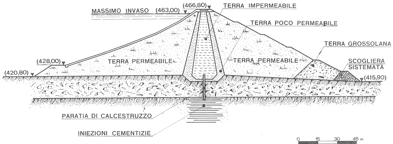
Sezione trasversale.
