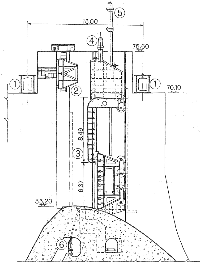
Fig. XX, 6. — Traversa PORTE DI FERRO (fiume Danubio). Sezione delle paratoie. 1, Travi della via di corsa della gru a portico ; 2, elemento della panconatura ; 3, paratoia doppia a gancio ; 4, servomotori a pistone dell'elemento superiore ; 5, servomotori a pistone dell'elemento inferiore ; 6, tubazione della insufflazione di aria contro la formazione di ghiaccio .
