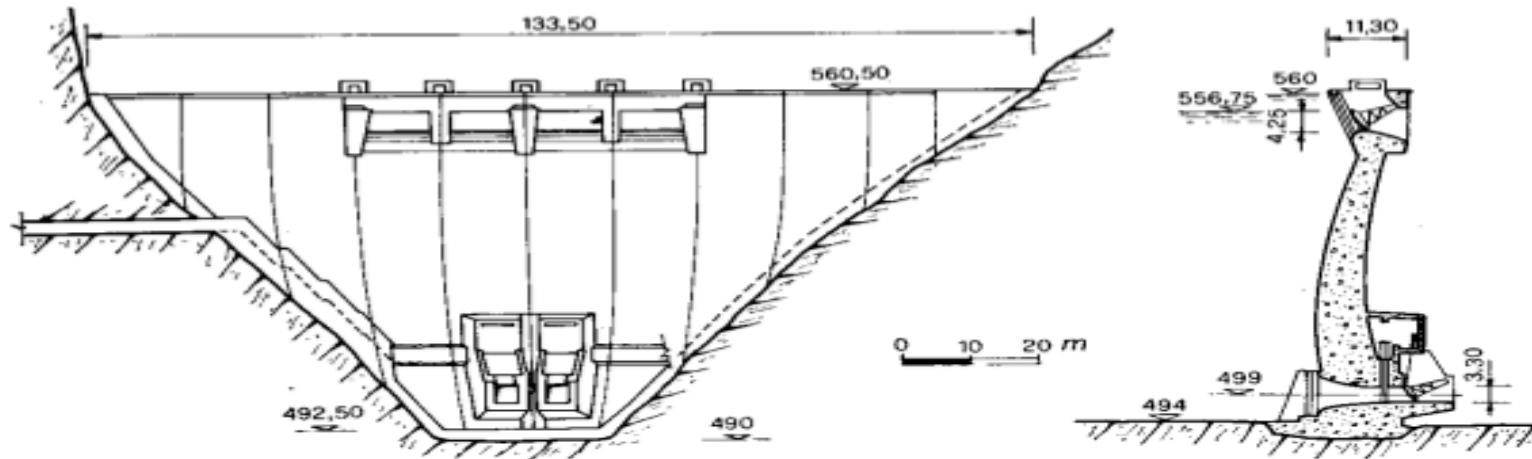
Fig. XVIII, 47. — Diga LA BARTHE sul fiume La Truyère (Francia). Altezza: m 71,50; sviluppo coronamento: m 133,50; capacità utile serbatoio: Mm^3 8; volume struttura: m^3 42.000. Quattro luci di sfioro di m 10 \times 4,25 dotate di paratoie a segmento. Capacità di scarico: m^3/sec 1800. Due scarichi di fondo in cunicoli blindati, dotati di paratoia piana di m 3,50 \times 3,50 e di paratoia a segmento di m 3,50 \times 3,30 . Capacità di scarico: m^3/sec 700. Vista da valle e sezione sugli scarichi.
