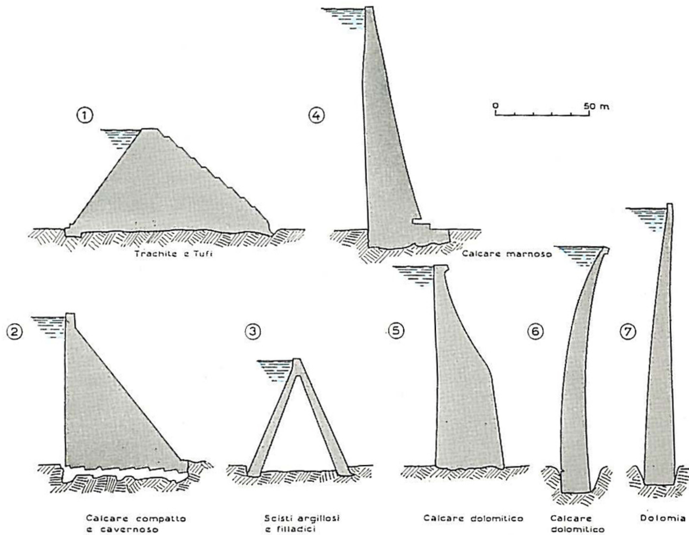
Fig. 398 - Principali tipi di dighe (in sezione trasversale).
