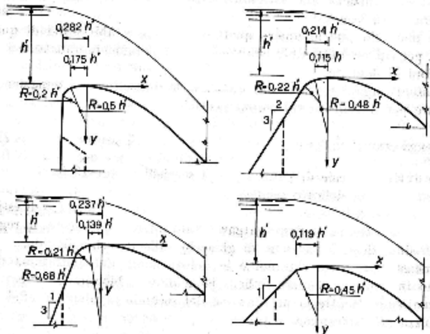
Fig. XVIII, 72. — Tipi di profili WES delle soglie sfioranti.
