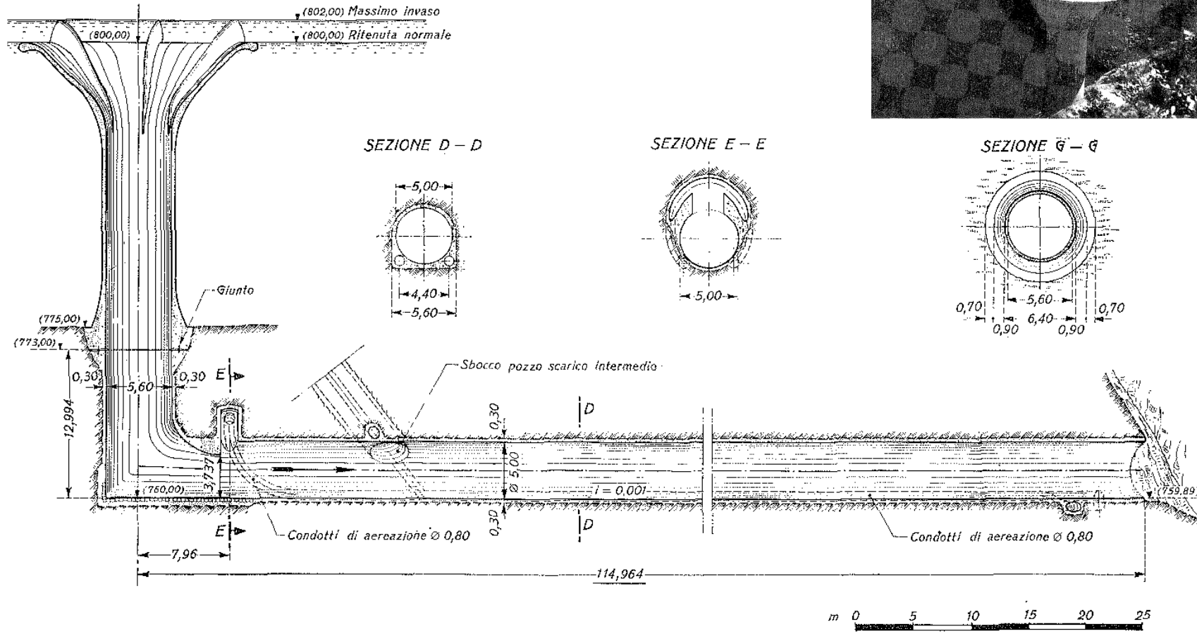
SEZIONE LONGITUDINALE A - A
