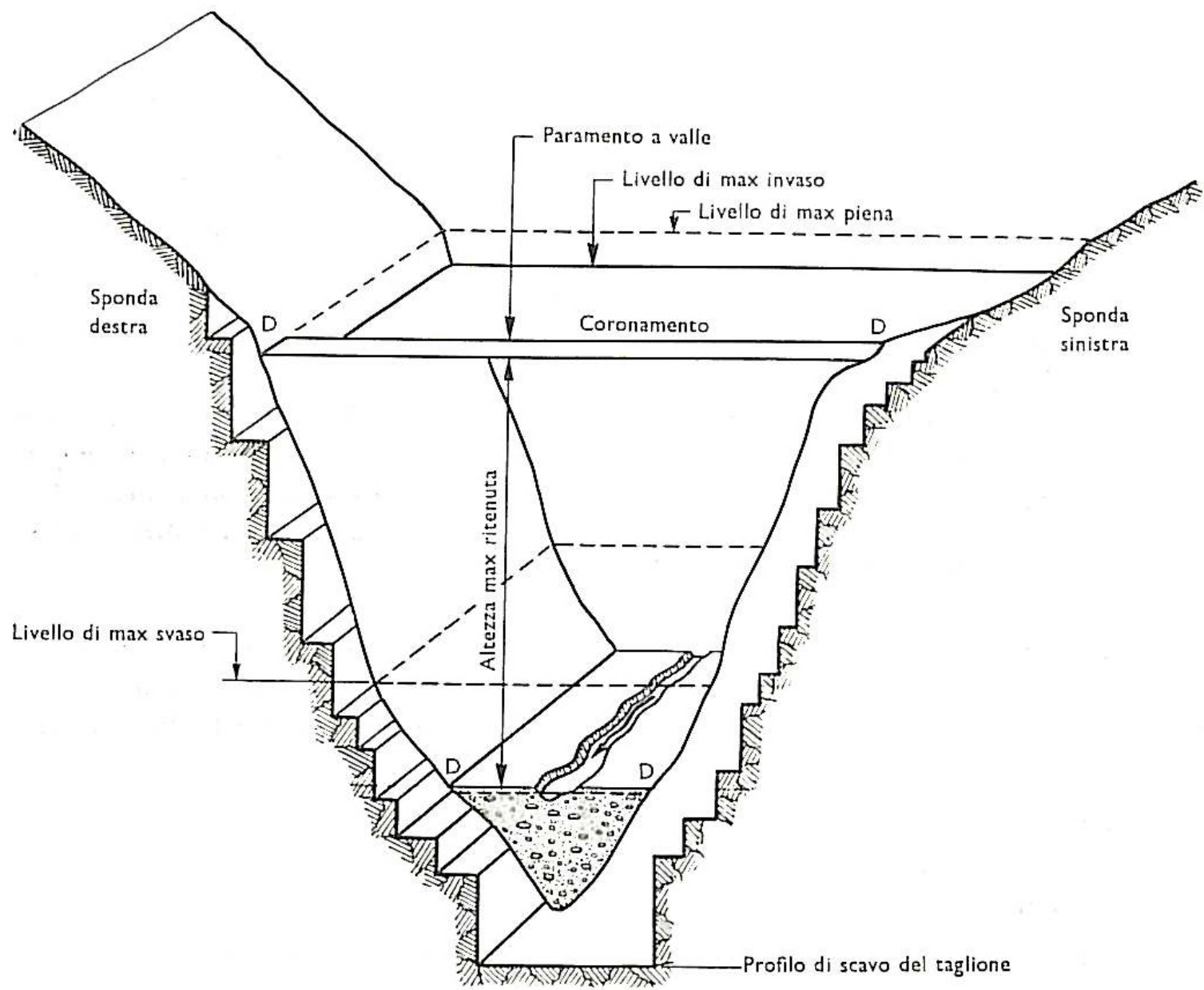
Fig. 400 – Nomenclatura essenziale relativa ad una diga di ritenuta.
