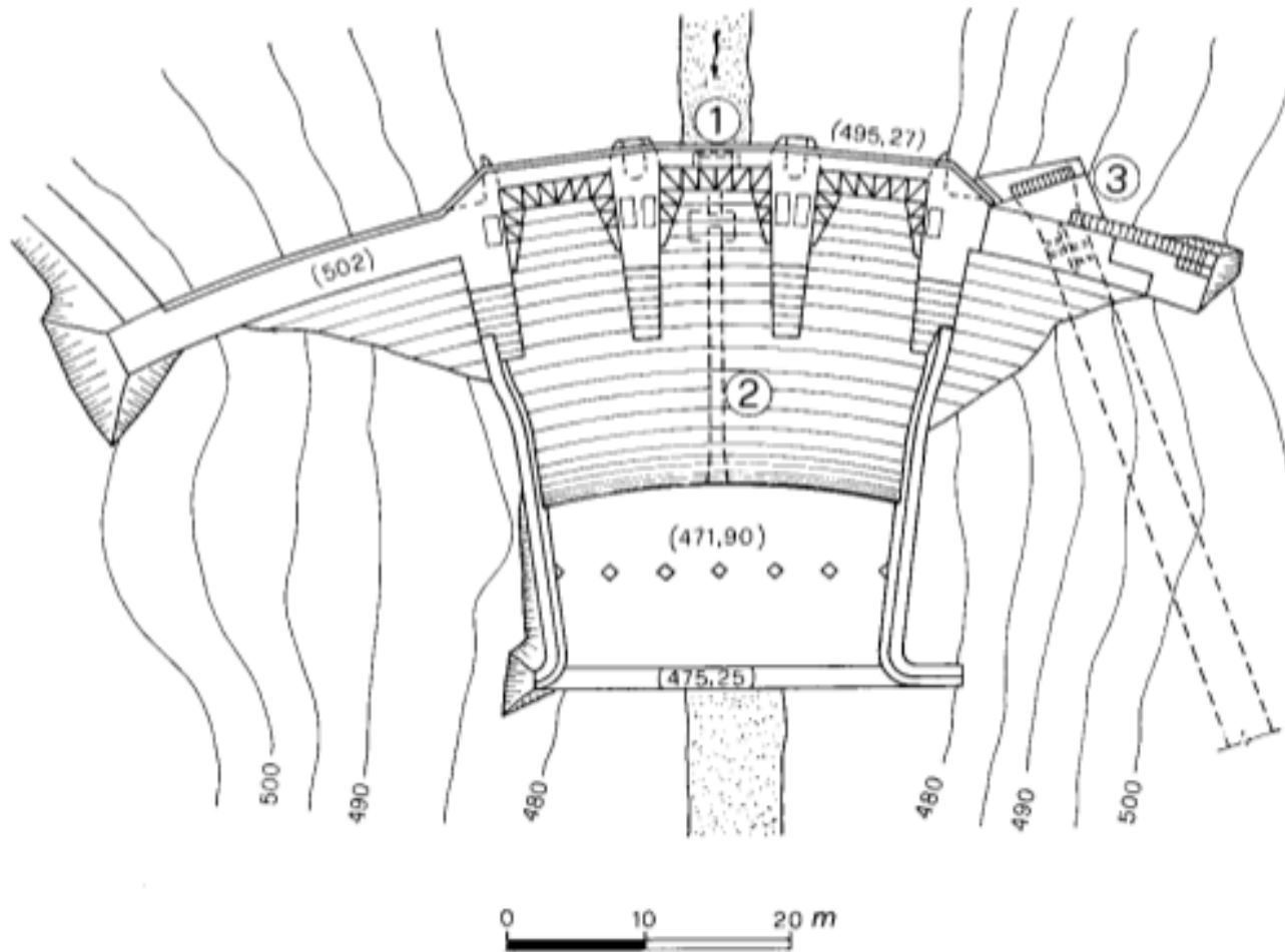
Fig. XVIII, 38. — Diga GAMMAUTA sul fiume Sosio (Sicilia) a gravità tracimabile. Anno fine costruzione: 1938; altezza: m 35; sviluppo coronamento: m 100; capacità totale serbatoio: Mm^3 2; volume struttura: m^3 31.000. Tre luci sforanti di m 8,50 \times 4,73 dotate di paratoie a segmento. 1, Imbocco scarico di fondo; 2, cunicolo di scarico di fondo; 3, opera di presa.
