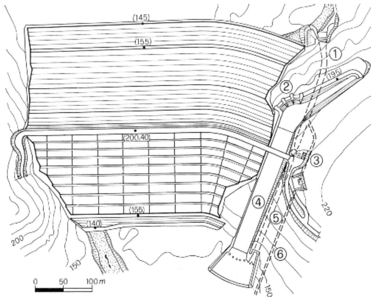
Fig. XVIII, 39. — Diga Occhito sul fiume Fortore (Puglia) (vedi fig. XV, 32). 1, Imbocco galleria di scarico di fondo; 2, sfiatore di superficie: soglia libera di m 112,49 di sviluppo e tre luci munite di paratoie a ventola di m 12,79 × 3, capacità totale di scarico 2100 m 3 /sec; 3, cabina di manovra delle valvole dello scarico di fondo; 4, scivolo dello scarico di superficie; 5, galleria di scarico di fondo diametro m 8,50; 6, galleria di derivazione.
