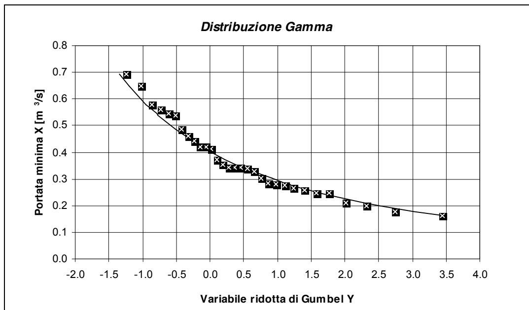
Figura 38 Adattamento della distribuzione Gammal alla serie dei minimi annui delle portate mensili.
