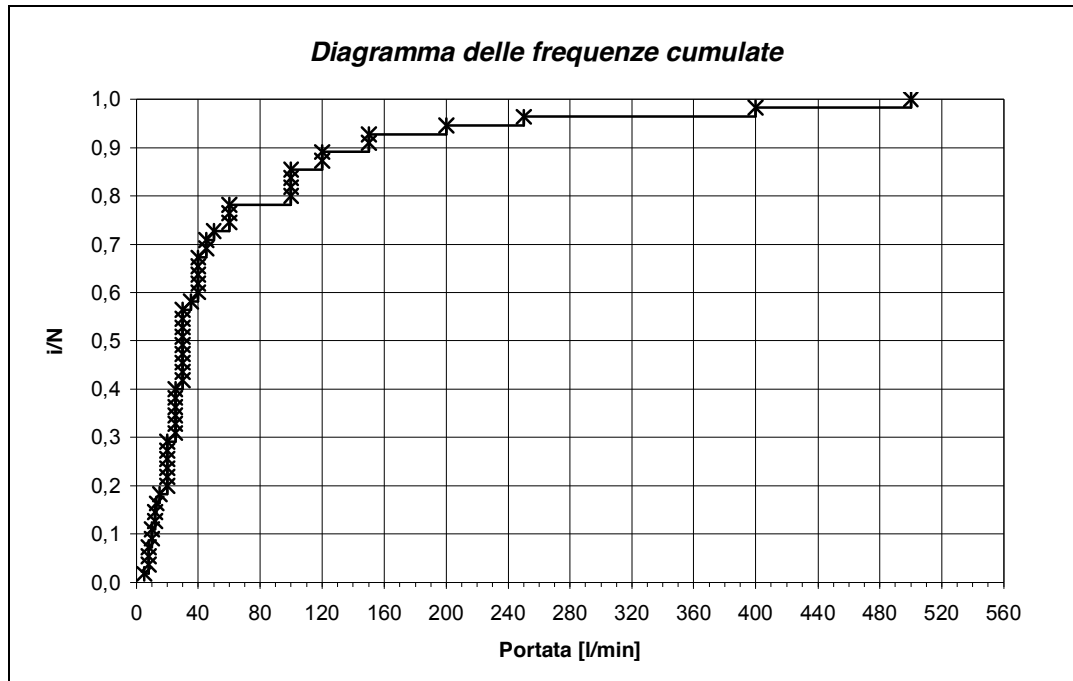
Figura 12 Diagramma delle frequenze cumulate delle portate delle sorgenti.
