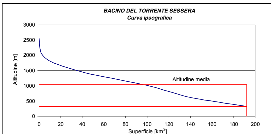
Figura 2 Curva ipsografica.
