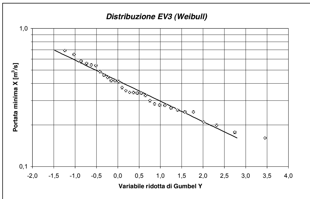
Figura 37 Adattamento della distribuzione di Weibull alla serie dei minimi annui delle portate mensili.
