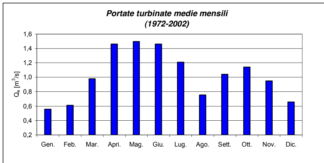
Figura 31 Grafico della portata turbinata media mensile.
