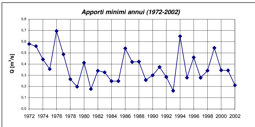
Figura 35 Andamento degli apporti minimi annui (1972-2002).
