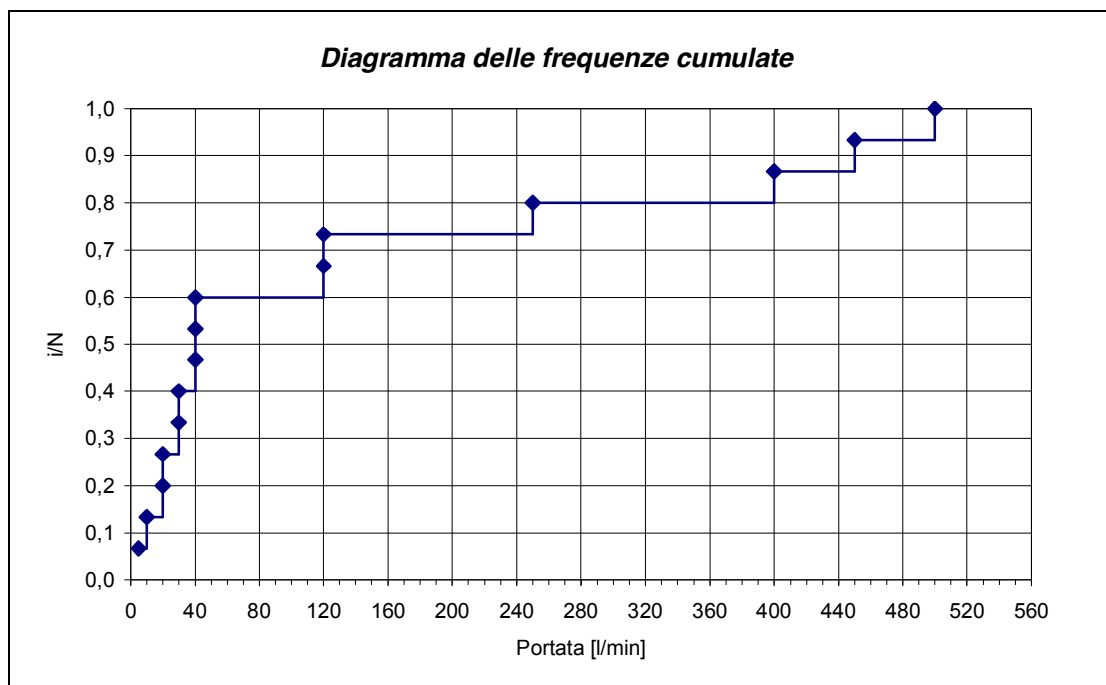
Figura 50 Diagramma delle frequenze cumulate delle portate delle sorgenti
