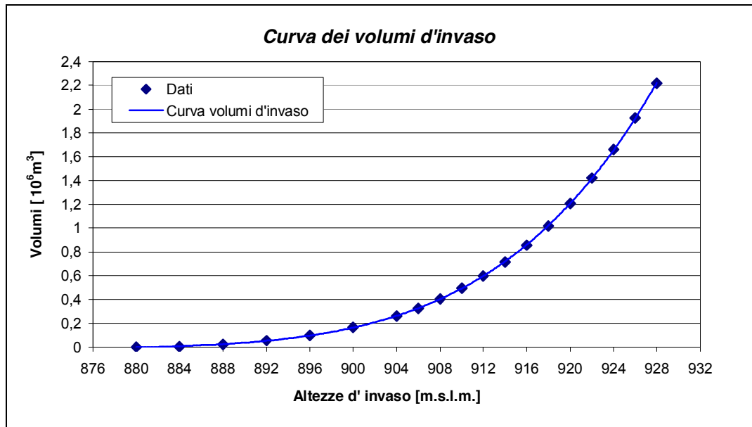
Figura 32 Grafico della curva dei volumi d'invaso.
