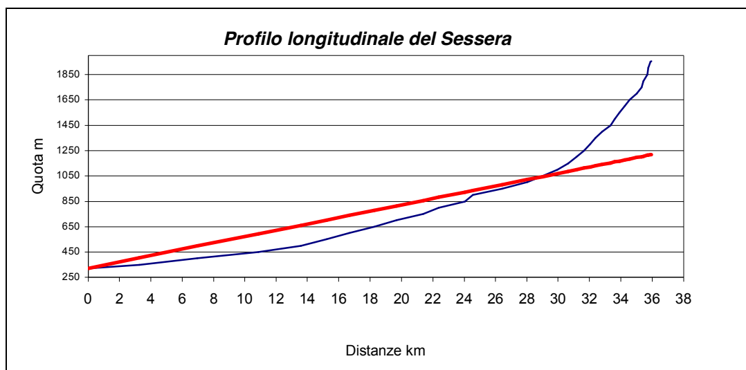
Figura 3 Profilo longitudinale dell'asta principale del torrente Sessera.
