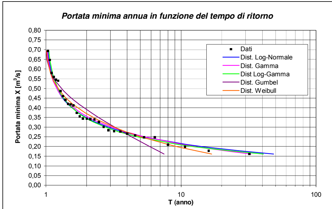
Figura 41 Legame tra la portata minima e il tempo di ritorno.
