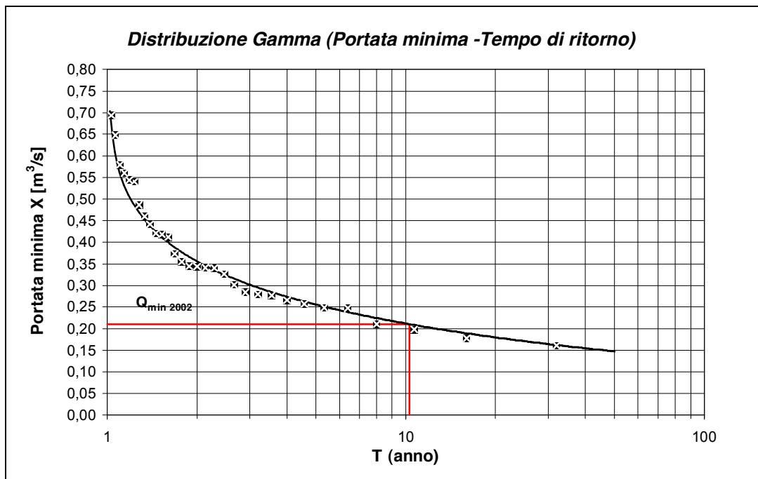
Figura 42 Legame tra portata minima e tempo di ritorno (Dist. Gamma).
