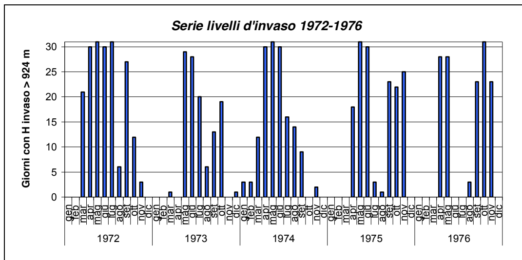
Figura 33 Serie livelli d'invaso 1972-1976.
