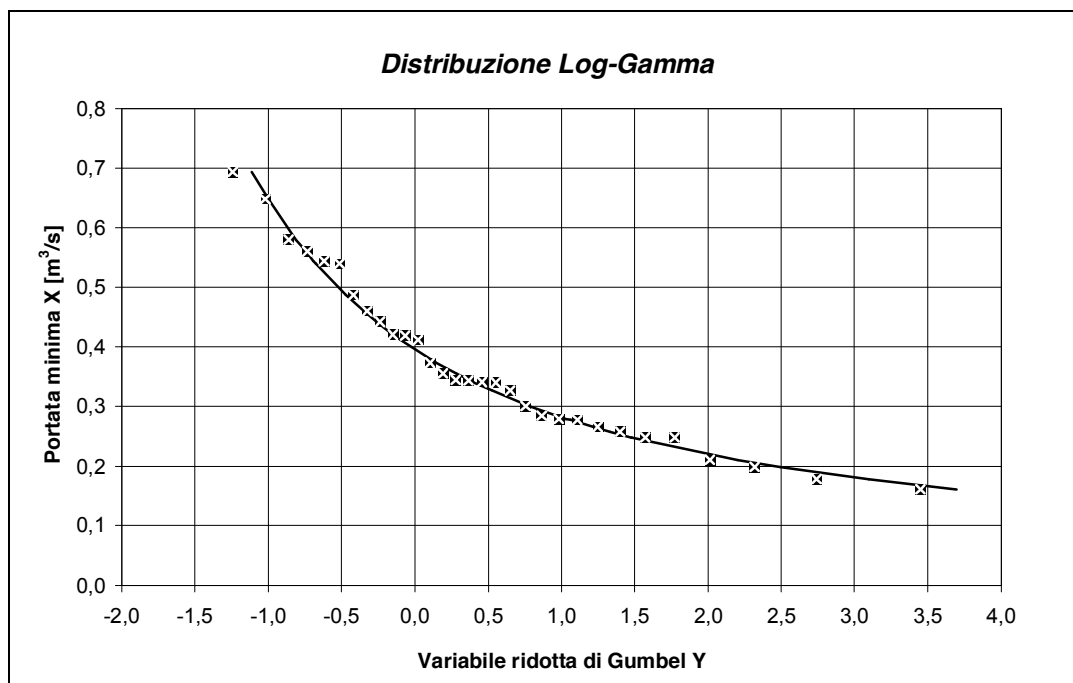
Figura 40 Adattamento della distribuzione Log-Gamma alla serie dei minimi annui delle portate mensili.
