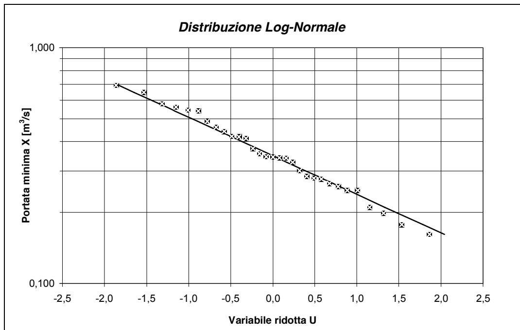
Figura 39 Adattamento della distribuzione Log-Normale alla serie dei minimi annui delle portate mensili.
