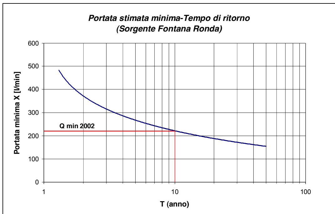
Figura 44 Legame tra portata minima stimata e tempo di ritorno (Fontana Ronda).
