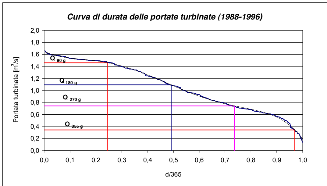
Figura 49 Curva di durata (1998-1996).
