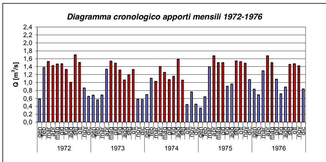
Figura 34 Grafico degli apporti mensili 1972-1976.
