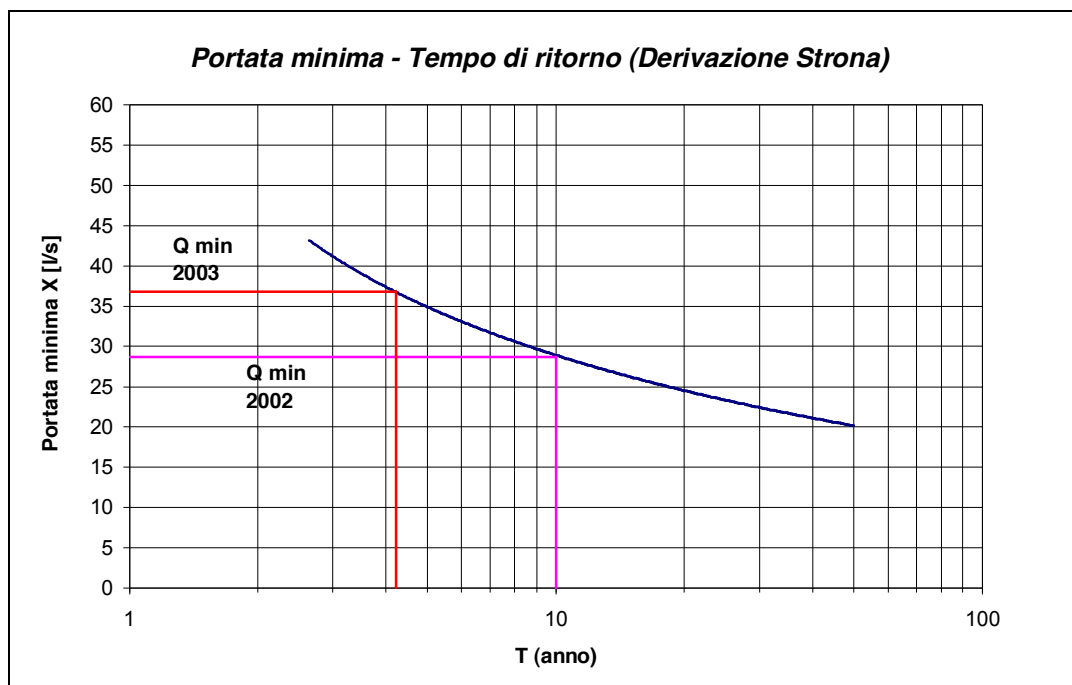
Figura 43 Legame tra la portata minima stimata e il tempo di ritorno (Strona).
