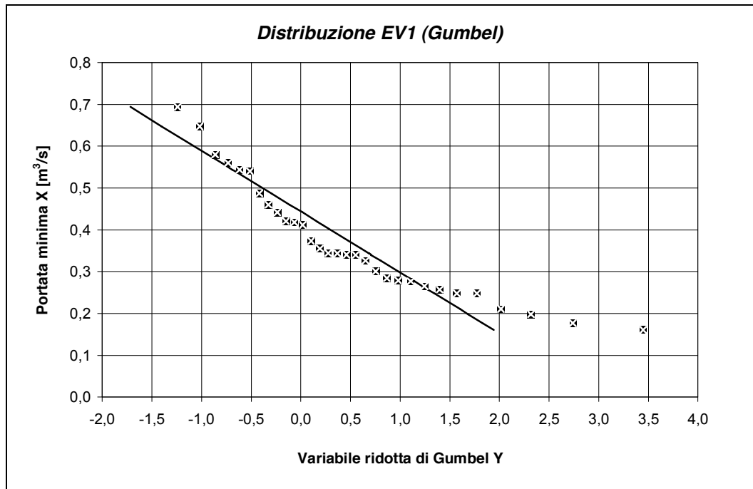
Figura 36 Adattamento della distribuzione di Gumbel alla serie dei minimi annui delle portate mensili.
