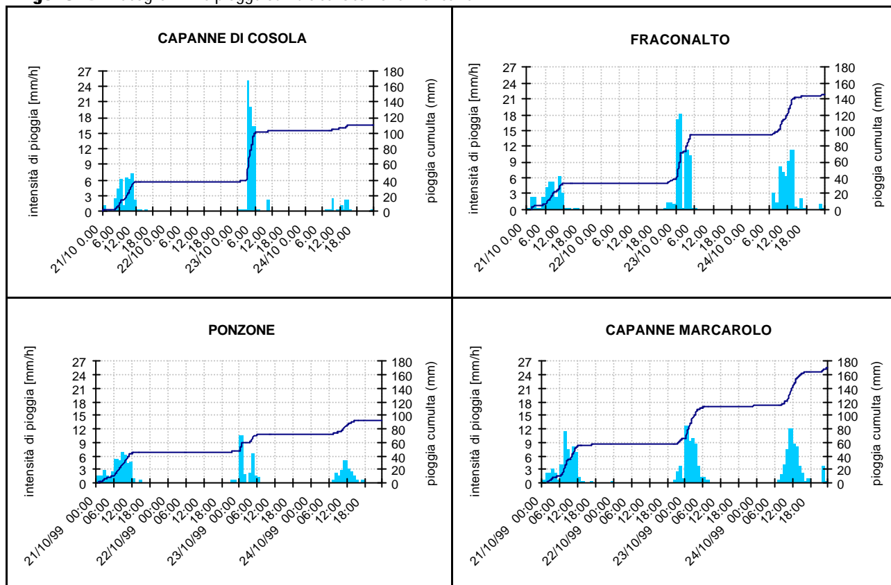
Figura 4 – letogrammi e piogge cumulate: stazione montane
