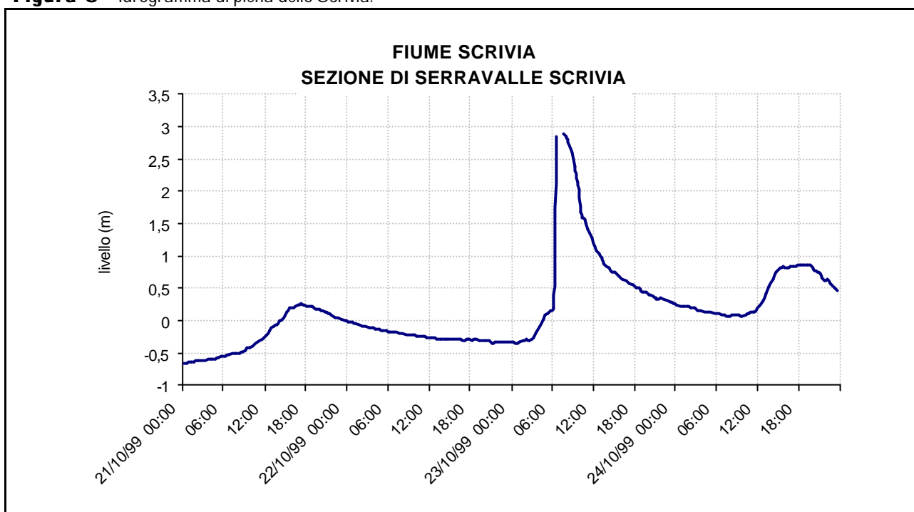
Figura 6 – Idrogramma di piena dello Scrivia.
