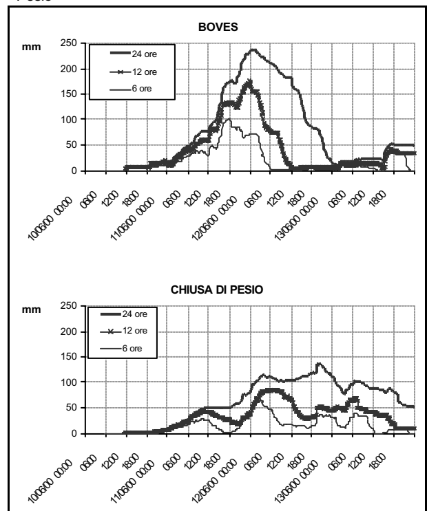
Figura 21 - Andamento delle precipitazioni cumulate in Val Pesio
