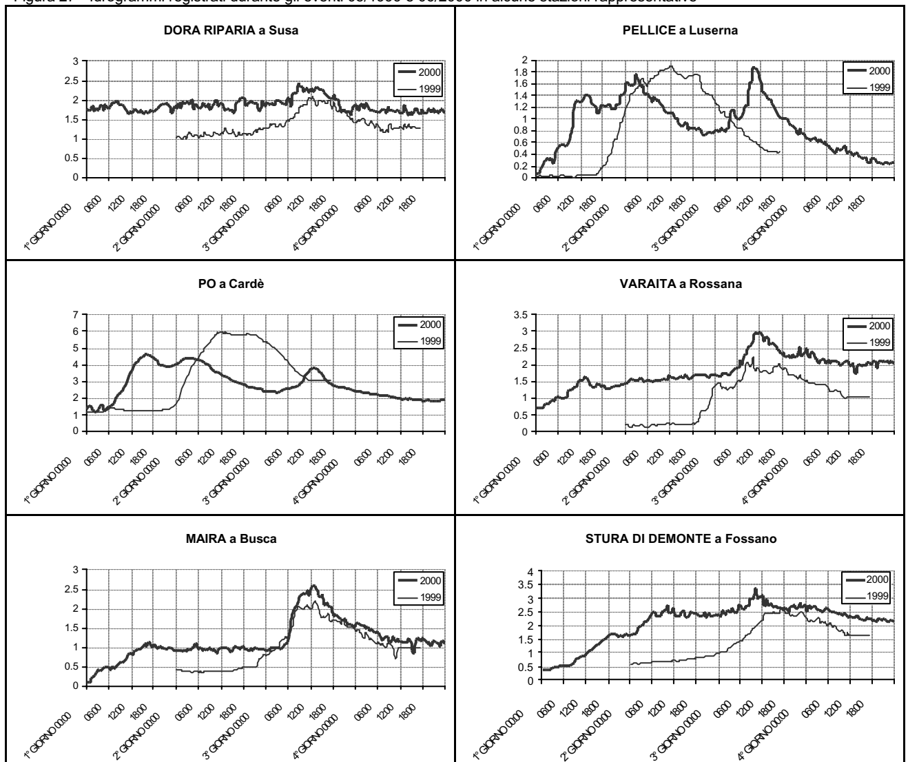
Figura 27 - Idrogrammi registrati durante gli eventi 05/1999 e 06/2000 in alcune stazioni rappresentative
