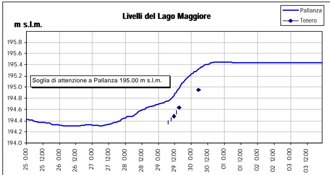
Figura 14 - Livelli del Lago Maggiore nei giorni dal 25 giugno al 3 luglio 1997
