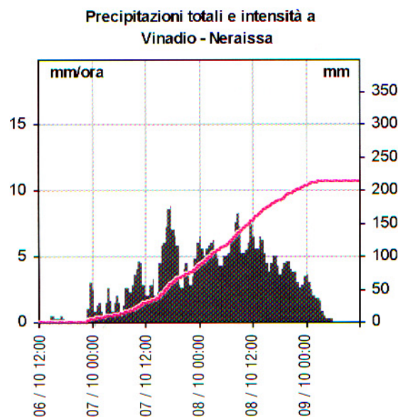
Fig. 3. Precipitazioni totali ed intensità oraria in alcune stazioni di misura.
