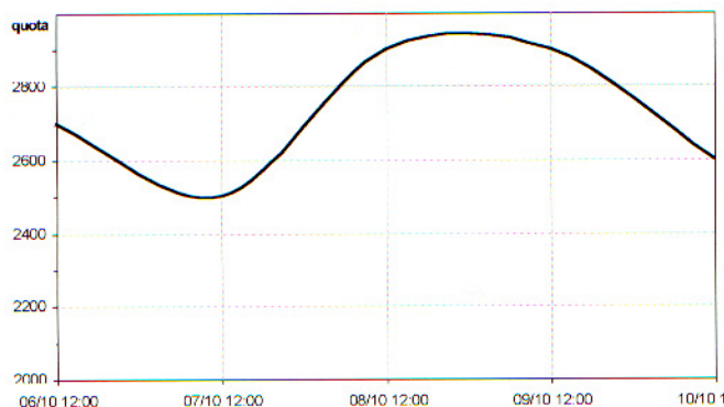
Fig. 1. Andamento dello zero termico nei giorni 6-10 ottobre 1996.
