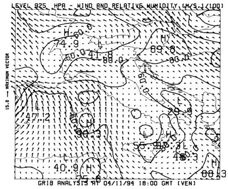
Fig. 6. Analisi ECMWF del campo di vento (m/s) e di umidità relativa (%) il giorno 4 alle ore 18 UTC ai livelli 500, 700, 850, 925 hPa.
