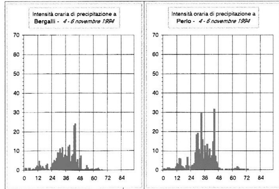
Fig. 32. Confronto tra eventi nel Piemonte meridionale.
