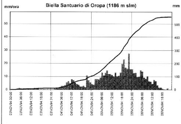
Fig. 30. Precipitazioni cumulate ed intensità orarie nei giorni 2-7 novembre 1994 in stazioni del Canavese (Lanzo e Meugliano) e del Biellese (Biella).
