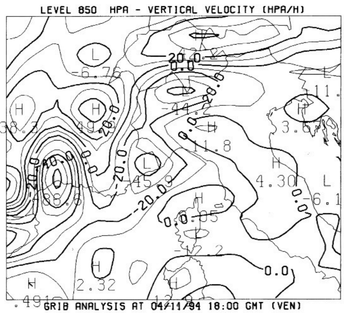
Fig. 7. Analisi ECMWF del campo di velocità verticale (hPa/h) il giorno 4 alle ore 18 UTC ai livelli 300, 500, 700, 850 hPa.
