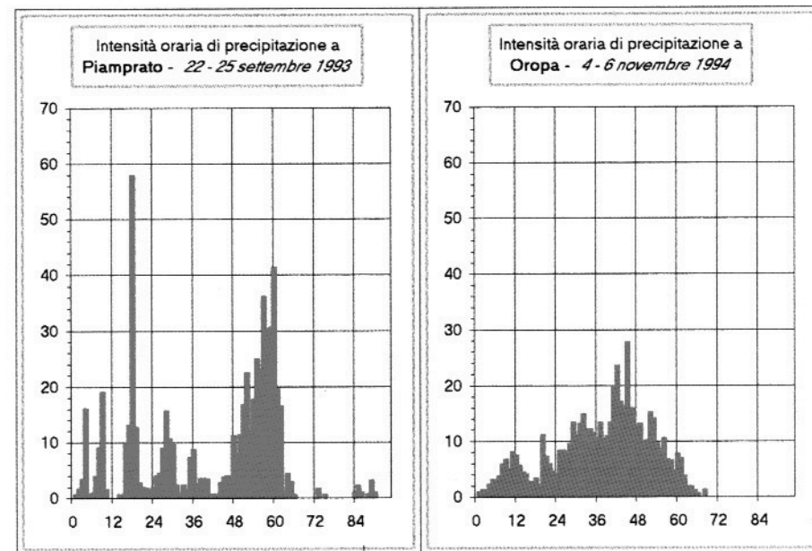
Fig. 34. Confronto tra eventi nel Piemonte settentrionale.
