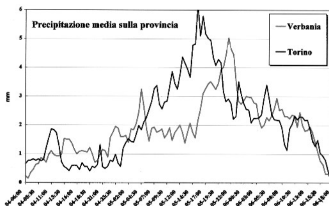
Fig. 18. Andamento temporale della precipitazione mediata sulle stazioni delle province di Verbania e Torino.
