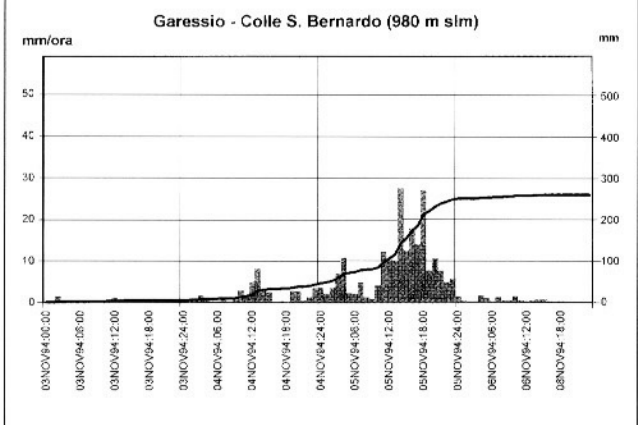
Fig. 29. Precipitazioni cumulate ed intensità orarie nei giorni 2-7 novembre 1994 in stazioni della Valle Tanaro (Perlo e Garessio).
