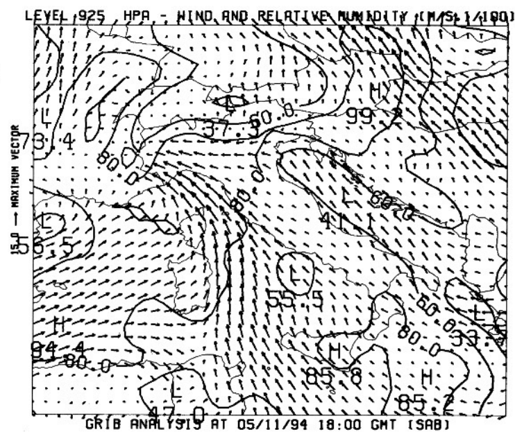
Fig. 9. Analisi ECMWF del campo di vento (m/s) e di umidità relativa (%) a 925hPa del 5 alle 00 UTC, 5 alle 06 UTC, 5 alle 12 UTC, 5 alle 18 UTC.
