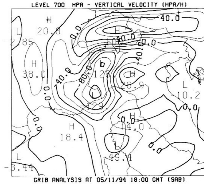
Fig. 14. Analisi ECMWF del campo di velocità verticale (hPa/h) a 700hPa del 5 alle 00 UTC, il 5 alle 06 UTC, il 5 alle 12 UTC, il 5 alle 18 UTC.
