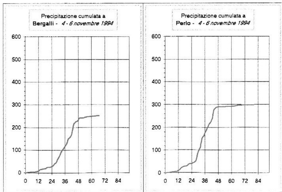
Fig. 31. Confronto tra eventi nel Piemonte meridionale.
