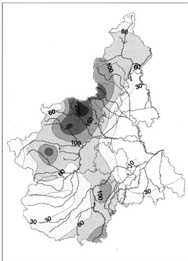
Fig. 22. Precipitazioni osservate cumulate dal 5 ore 12 UTC al 6 ore 00 UTC, isolinee a 2 mm, 5 mm, 10 mm, 30 mm, 60 mm, 100 mm, 150 mm, 200 mm.
