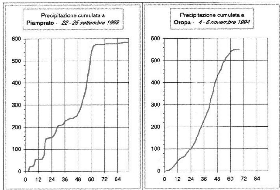
Fig. 33. Confronto tra eventi nel Piemonte settentrionale.
