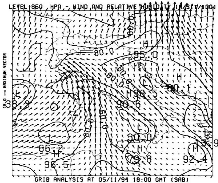
Fig. 8. Analisi ECMWF del campo di vento (m/s) e di umidità relativa (%) a 850hPa del 5 alle 00 UTC, 5 alle 06 UTC, 5 alle 12 UTC, 5 alle 18 UTC.
