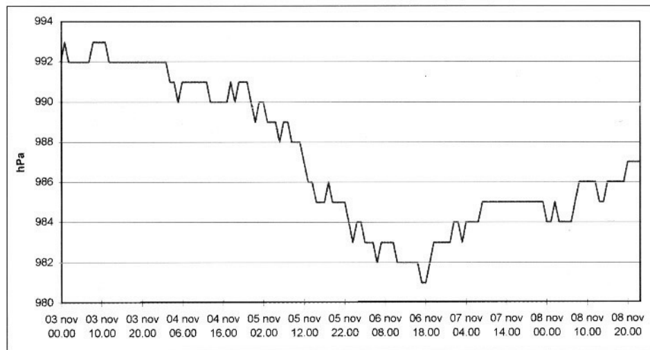
Fig. 26. Andamento della pressione al livello della stazione di Alessandria.
