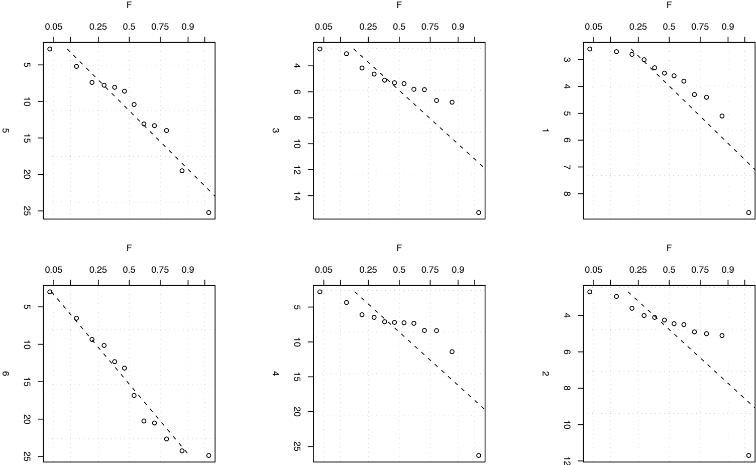
Figura F.22: Normal plot dei deflusi minimi mensili, bimestrali, ..., semestrali. (30/37 Bormida a Cassine)
