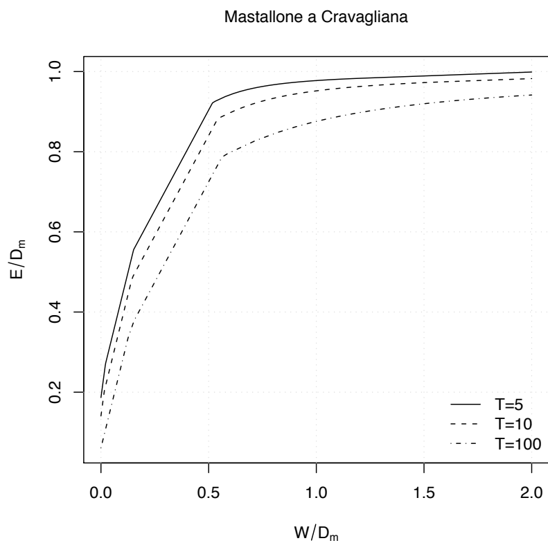
Figura F.35: Curve adimensionali di possibilità di regolazione per gli invasi in progetto (2/3).
