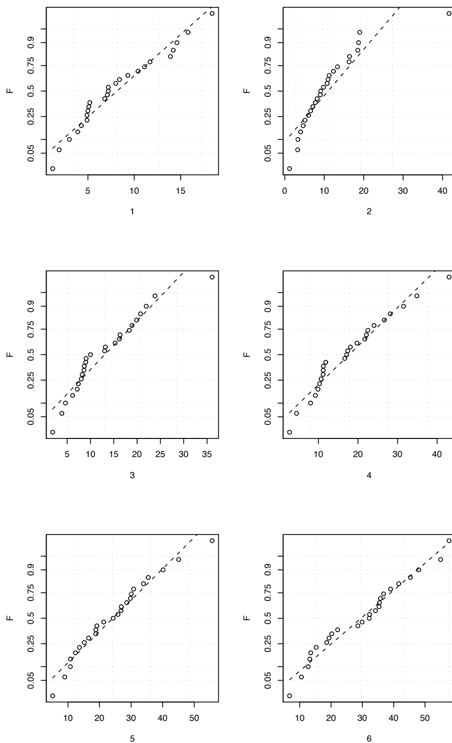
Figura F.22: Normal plot dei deflussi minimi mensili, bimestrali, ..., semestrali. (28/37 Scivia a Serravalle)
