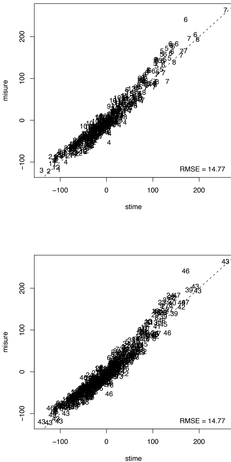
Figura F.9: Diagrammi diagnostici per le Serie di Fourier di Paragrafo 7.2.1. Nella figura in alto i numeri indicano i mesi dell'anno, in quella in basso il codice delle stazioni; in basso a destra è indicato l' RMSE_{reg} medio.
