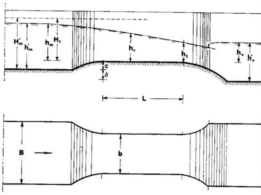
Fig. 2. — Schema di funzionamento di un venturimetro per canali.
