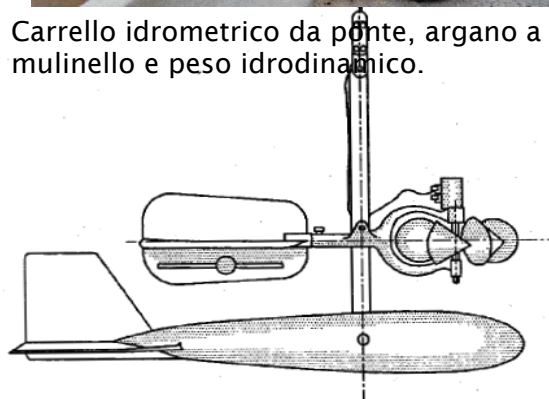
Fig. 5.8 Pesce con mulinello ad asse verticale (Linsley et al. , 1949)
