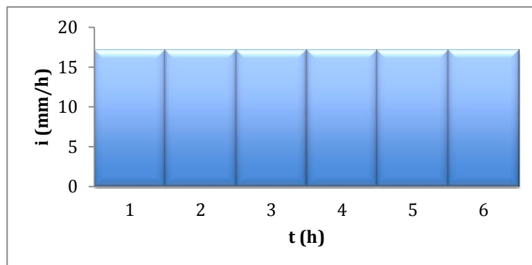
Fig. 2 – Ietogramma lordo costante
