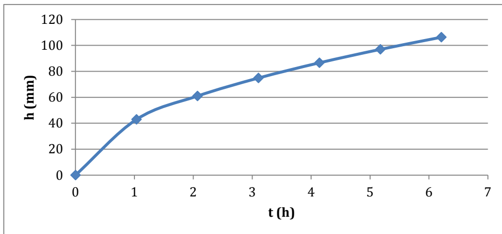
Fig. 1 – Curva di possibilità pluviometrica
