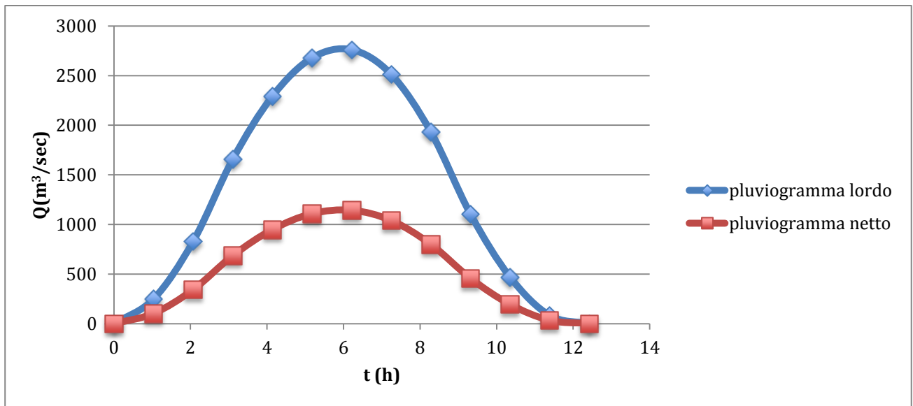
Fig. 4 - Pluviogrammi
