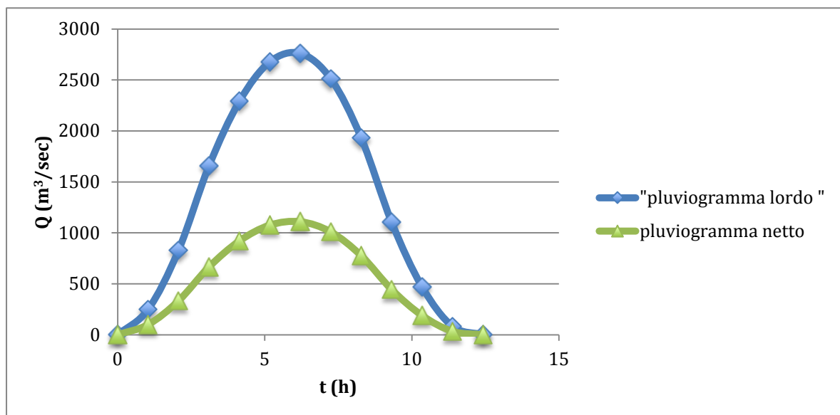
Fig. 3 – Pluviogrammi
