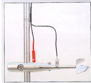
Misure con calata da ponte (mulinello + asta correntometrica)
