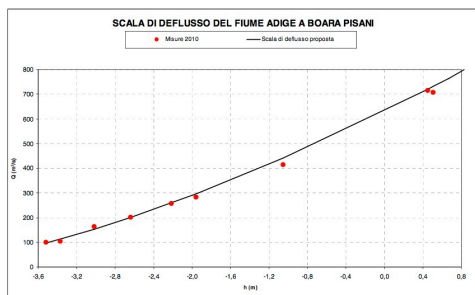
Figura 1 - Scala di deflusso proposta per il teleidrometro sul fiume Adige a Boara Pisani
