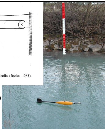
Misure da teleferica (mulinello zavorrato)
