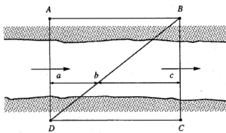
Fig. 5.20 Misura di velocità superficiale con il metodo del galleggiante
