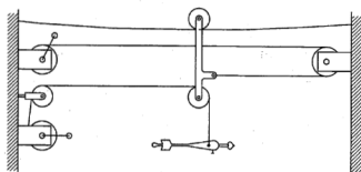
Fig. 5.12 Teleferica per le misure con il mulinello (Roche, 1963)
